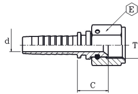
JIC FEMALE 37° FLARE WITH THRUST WIRE NUT FEMMINA JIC SV. 37° CON DADO SPINATO 041645
