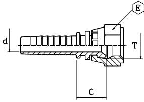
JIC FEMALE 37° FLARE FEMMINA JIC SV. 37° 041627
